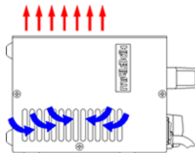
Горизонтальная установка
