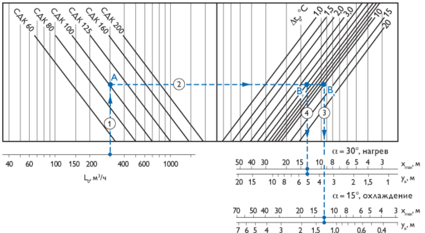
Номограмма 2. Расчет координат x_{\text{max}} и Y_B наклонной неизотермической струи при углах наклона \alpha = 15^\circ (рис. 1а) и \alpha = 30^\circ (рис.1б).
