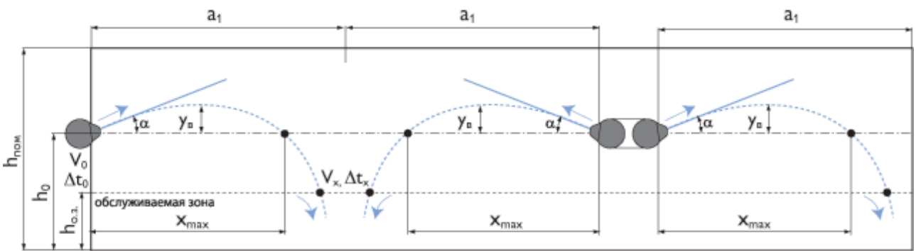
Рис.1. Траектория приточной струи при подаче по схеме Б:
